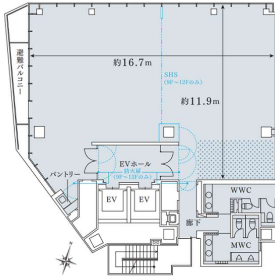
4F-12F(基準階)
