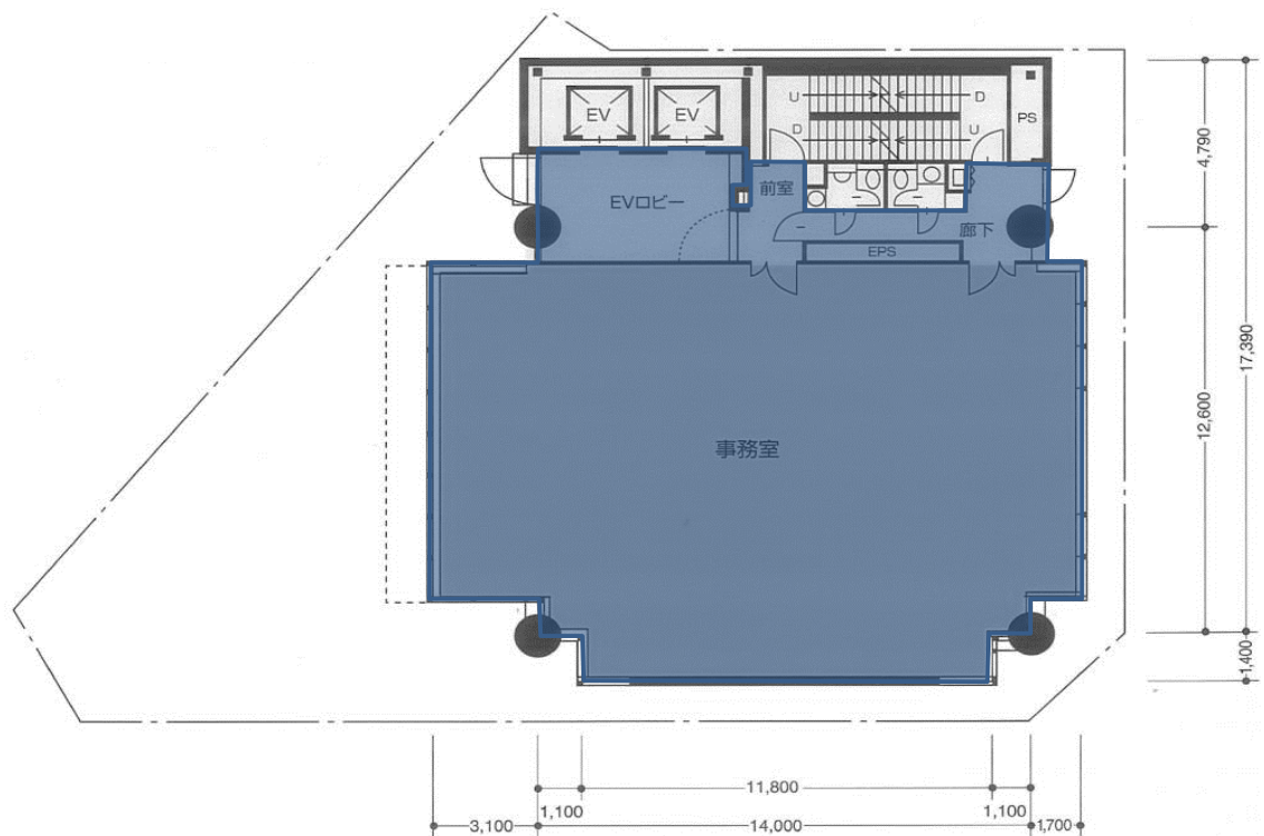
10階 平面図
